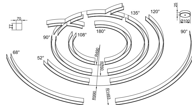
UGR optika
